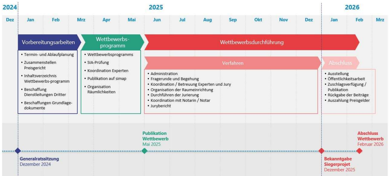
Abb. 21: Terminplan Verfahren
